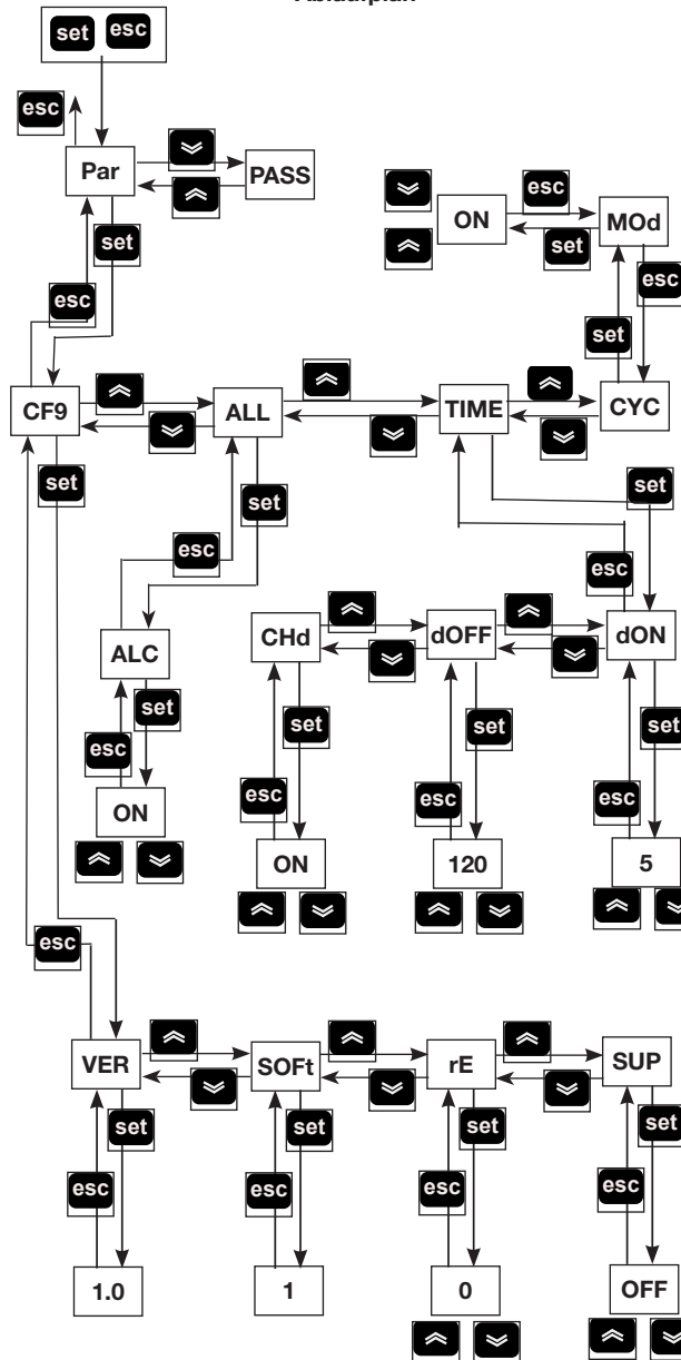
Ablaufplan
